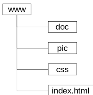
Рис. 1. Структура сайта
